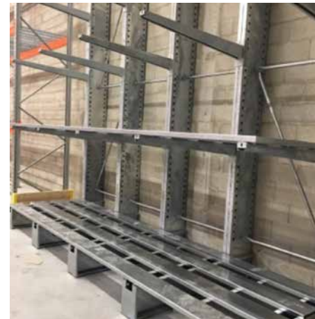
Platelage sur Cantilever
